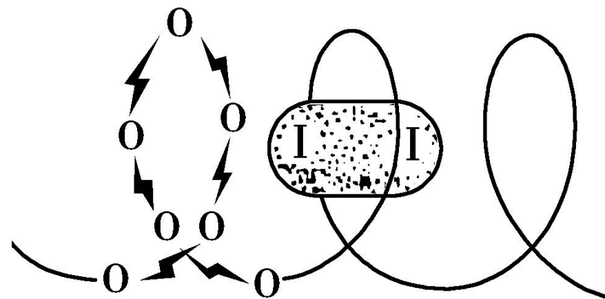
淀粉-碘蓝色物质结构示意图
