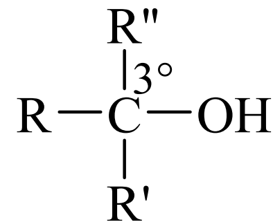
叔醇
