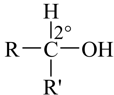
仲醇
