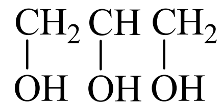
丙三醇
