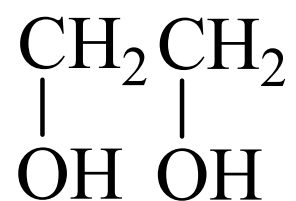
乙二醇
