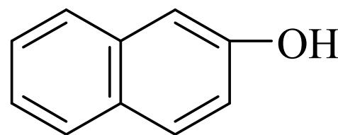
\beta -萘酚
