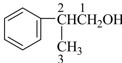
2-苯基-1-丙醇
