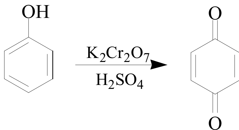
对苯醌
