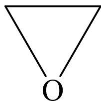
环氧乙烷
