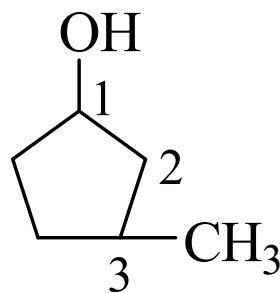
3-甲基环戊醇
