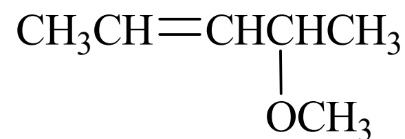
4-甲氧基-2-戊烯
