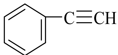
苯乙炔
