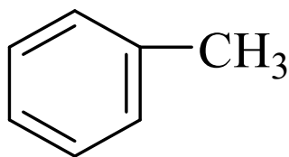
甲苯
