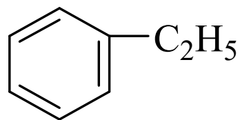
乙苯
