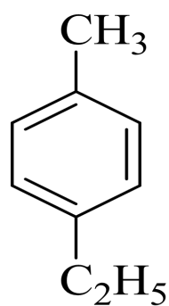
4-乙基甲苯
