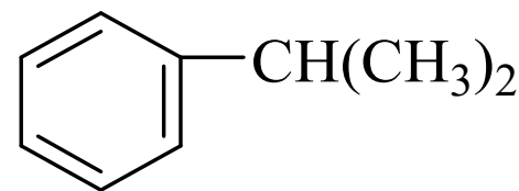
异丙苯
