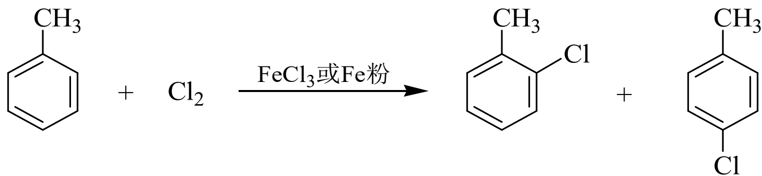
邻氯甲苯
