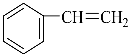
苯乙烯
