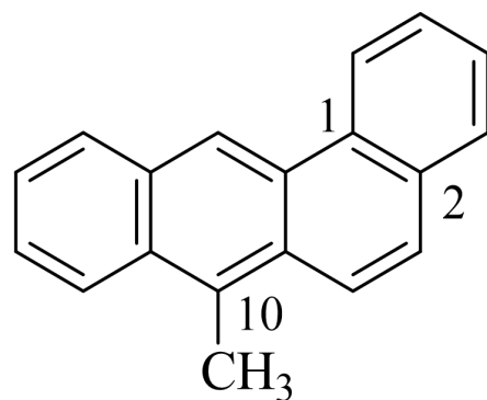
10-甲基-1,2-苯并蒽
