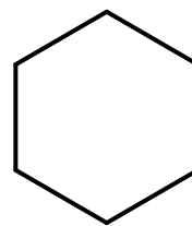
环己烷
