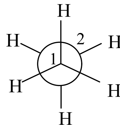
交叉式
